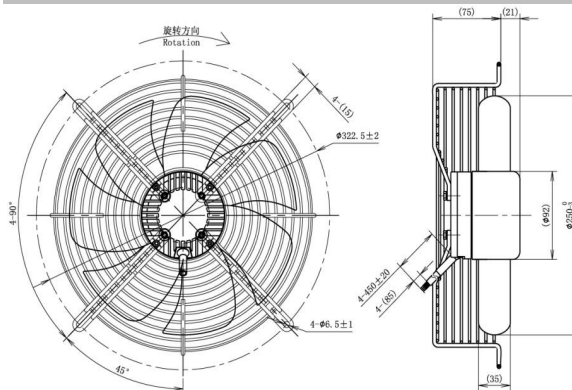
A1SE250C Cylinder Fan 带圆筒
