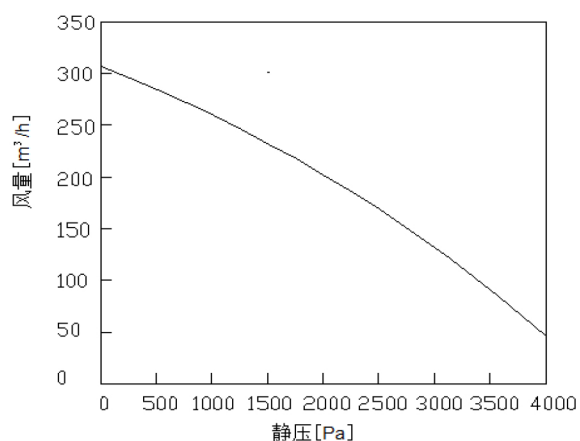
风机性能曲线
